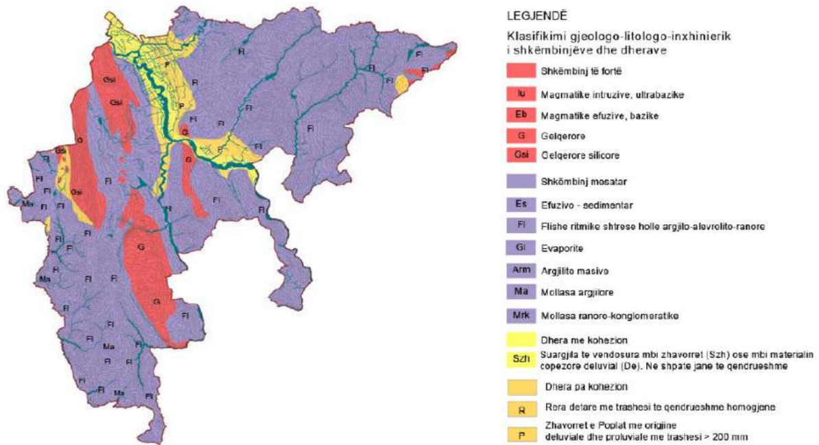
Figure 9. Harta gjeolojiko-inxhinierike e Bashkise Berat
