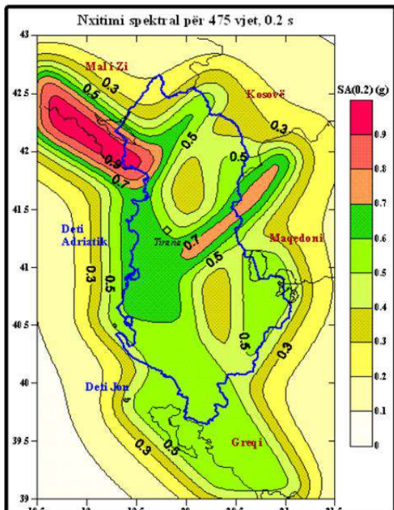
Figure 12. Harta e shpejtimit spektral SA (0.2) me shuarje 5% në truall shkëmbor dhe probabilitet 10%/50 vjet ose 475 vjet periodë përsëritje 475 (Majtas) dhe Harta e Rrezikut Sizmik në Shqipëri (Djathtas) (Burimi: Aliaj et al. 2010).
