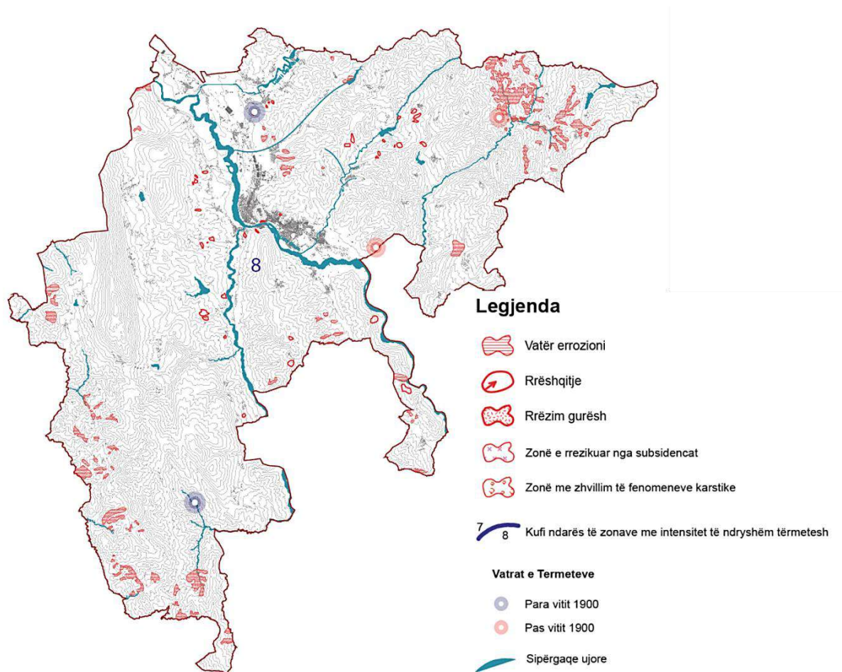
Figure 10. Harta e rrezikut gjeologjik ne Bashkine Berat
