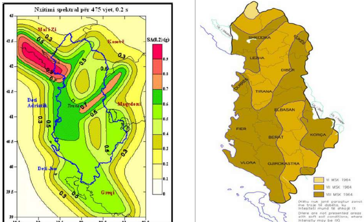
Figure 16. Harta e shpejtimit spektral SA (0.2) me shuarje 5% në truall shkëmbor dhe probabilitet 10%/50 vjet ose 475 vjet periodë përsëritje 475 (Majtas) dhe Harta e Rrezikut Sizmik në Shqipëri (Djathtas) (Burimi: Aliaj et al. 2010).
